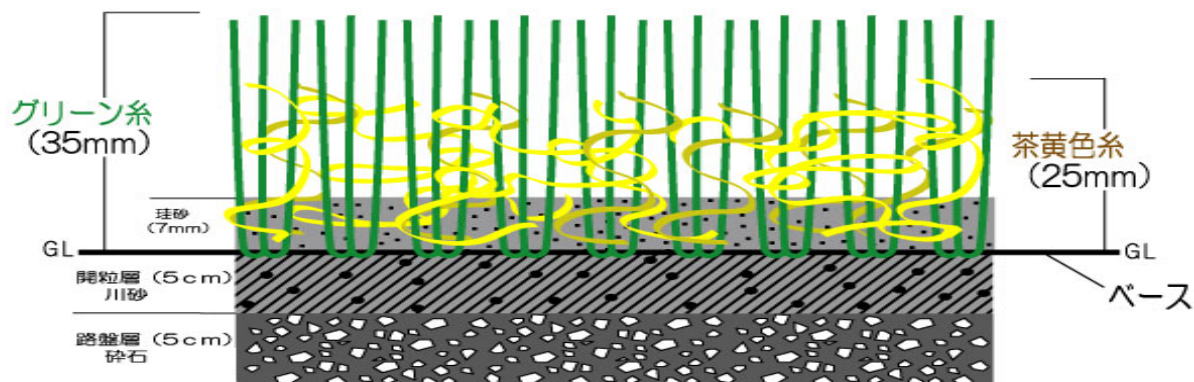
ステップターフ設計断面図 ( S T - R 3 5 )
